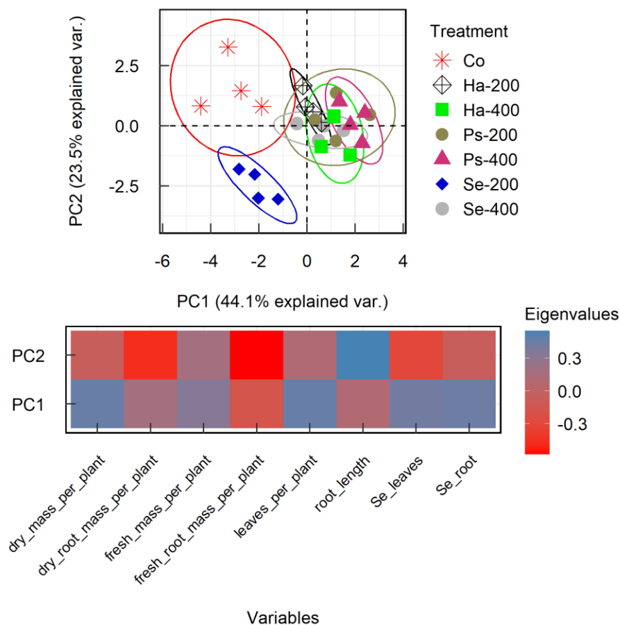
Slika 10. Analiza glavnih komponenata učinaka (Principal component analysis – PC) obrade na morfološke karakteristike i koncentracije selena u različitim dijelovima matovilca (gore) te varijabilni faktori (korelacije između PC-a i originalnih varijabli, dolje). Izvor: Galić, neobjavljeni rezultati (2024.)
