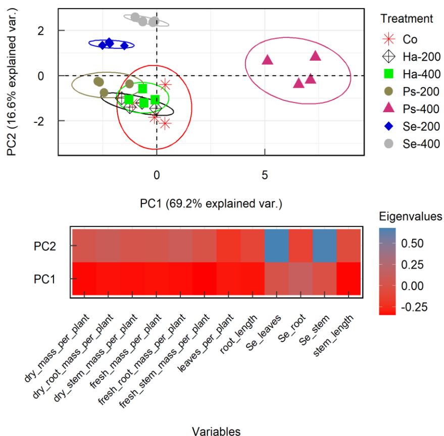
Slika 11. Analiza glavnih komponenata učinaka tretmana na morfološke karakteristike i koncentracije selenata u različitim dijelovima biljke kod amaranta (iznad) i opterećenja varijablama (korelacije između glavnih komponenata i izvornih varijabli, ispod). Izvor: Galić, neobjavljeni rezultati (2024.)
