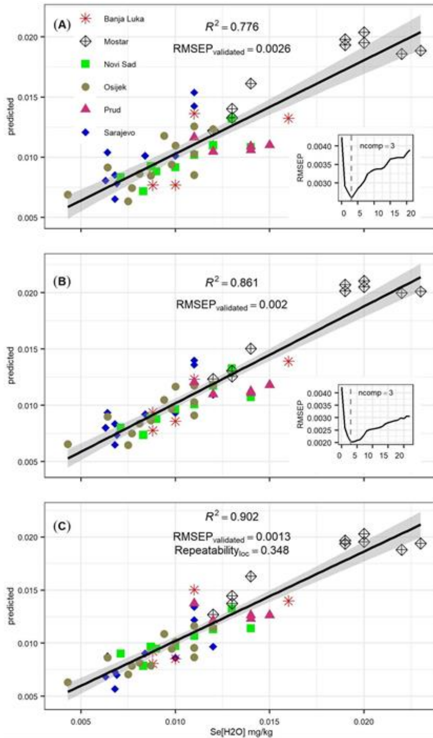
Slika 4. Model parcijalnih najmanjih kvadrata (PLS - partial least squares) regresije za \text{Se}_{\text{H}_2\text{O}} , uključujući svojstva tla i koncentracije drugih elemenata (A), \text{Se}_{\text{Tot}} (B) i PLS rezultate iz (B) zajedno s glavnim učinkom lokacije u mješovitom modelu (C). Odgovarajuće validacijske pogreške, odabrani broj komponenata i ponovljivost slučajnog učinka lokacije prikazani su unutar grafova. Izvor: Galić i sur. (2023.)
